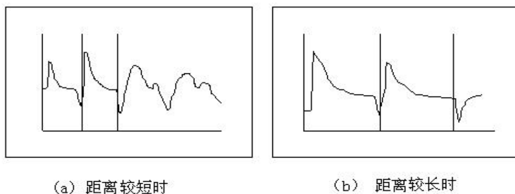
图 17 故障在测试终端波形
