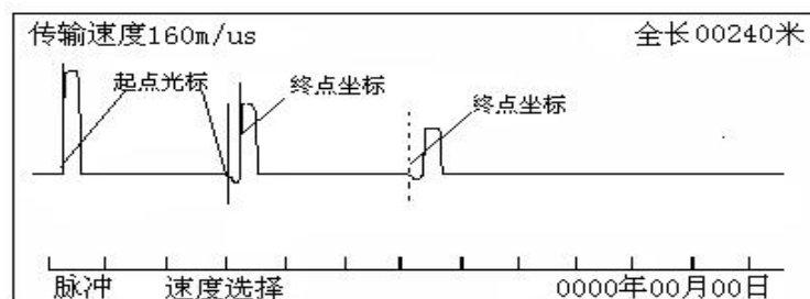
图 14 冲闪法电流取样测试波形
