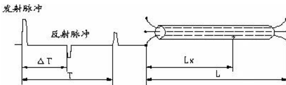
图 10 测试原理图
