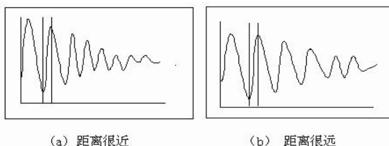
图 15 故障在测试始端波形
