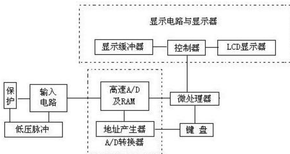
图 1 测试原理图
