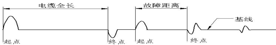
图 24 故障点二次击穿测试波形
