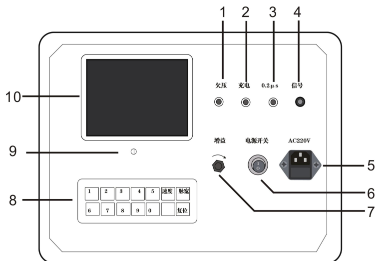
图 2 面板布局图
