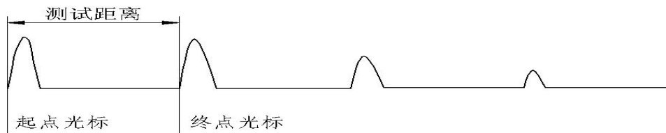
图 23 冲闪法测试纯短路故障波形
