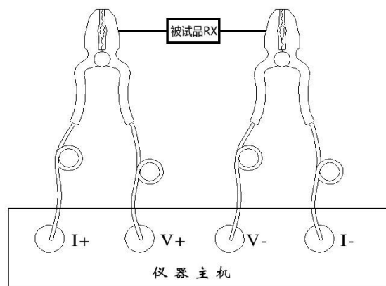
图二 接线图
