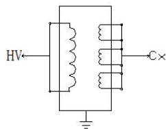
图 6-5 CT 接法
