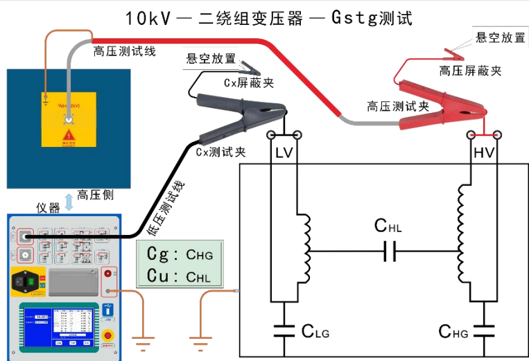
(1)、两绕组变压器 C_{HG}+C_{HL} 测试接线
