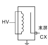
图 6-6 CT 接法
