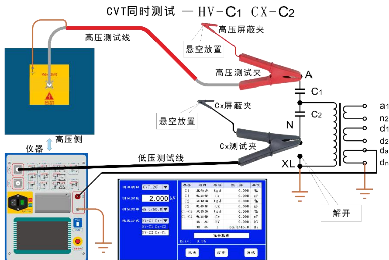
(5)、CVT 同时测试，上端有 C0 的测试（一次完成测试）
