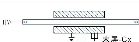
图 6-8 套管正接法
