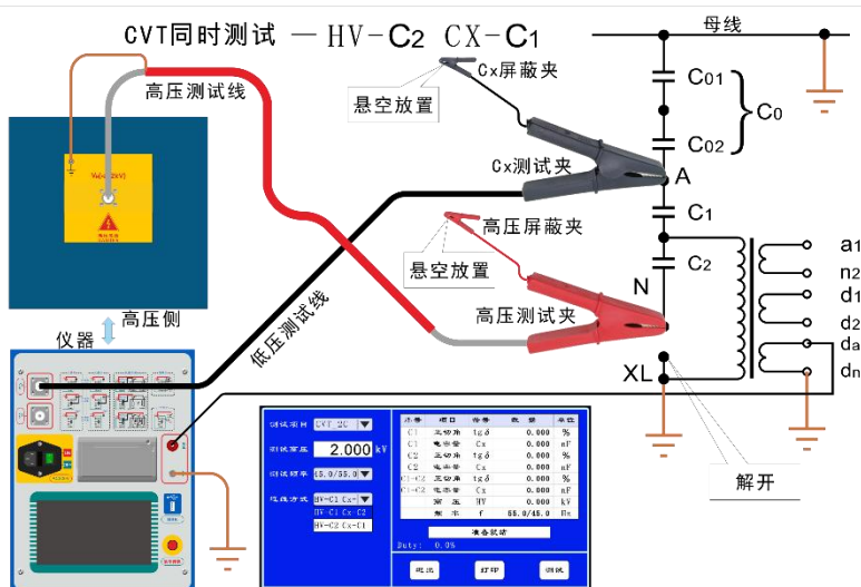
(6)、CVT 同时测试，上端有 C01 和 C02 的测试（一次完成测试）
