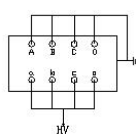
图 6-12 变压器反接法
