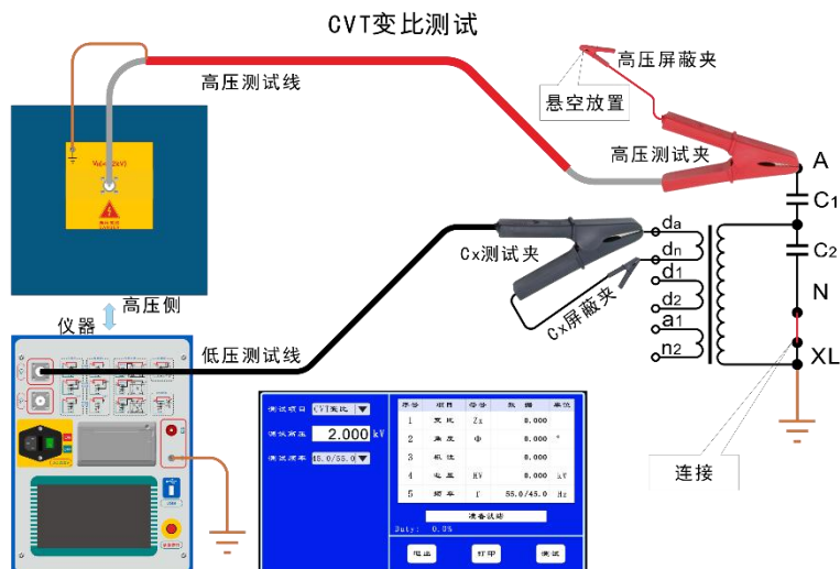
(1)、PT 变比测试
