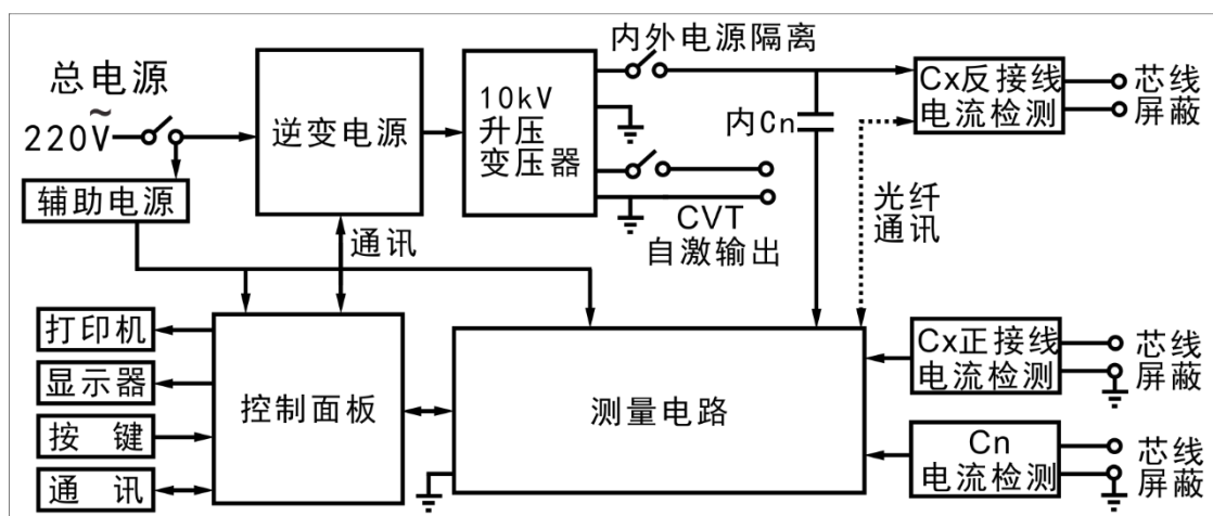
图 2—1 测量原理图
