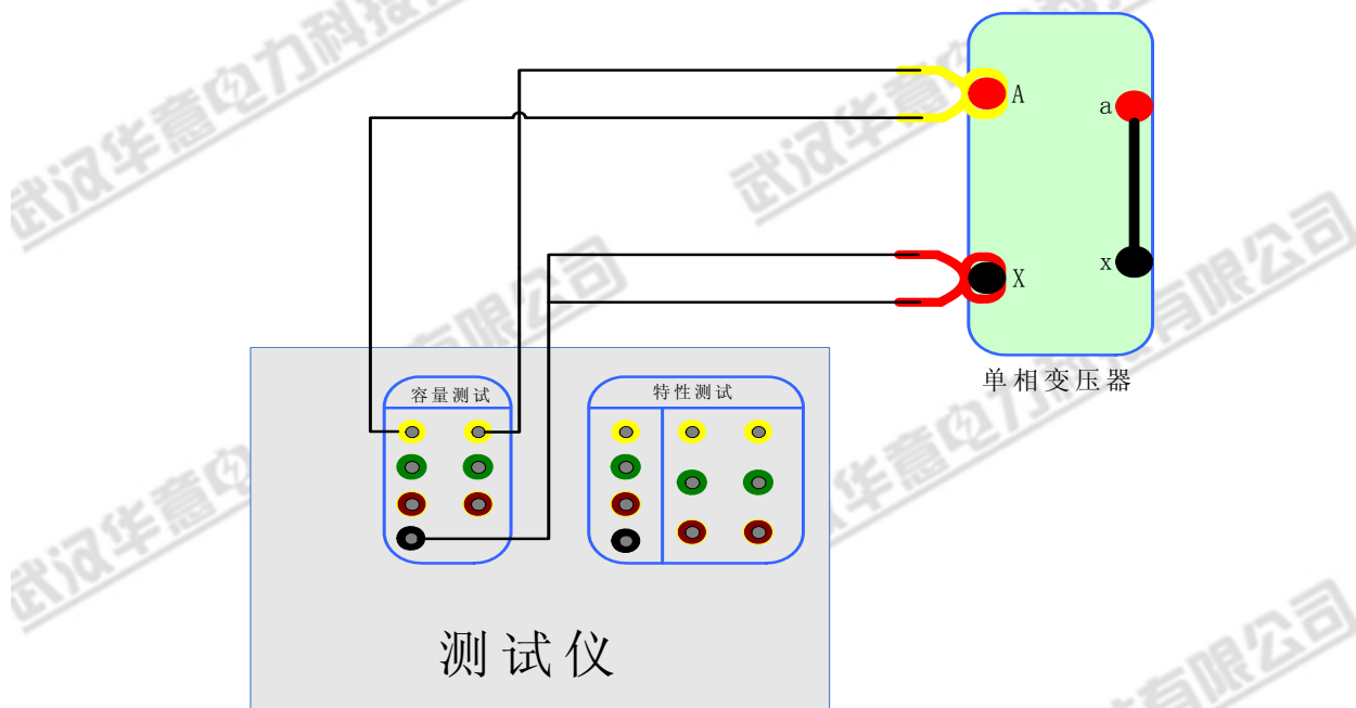
3. 双表法空载试验接线图:
