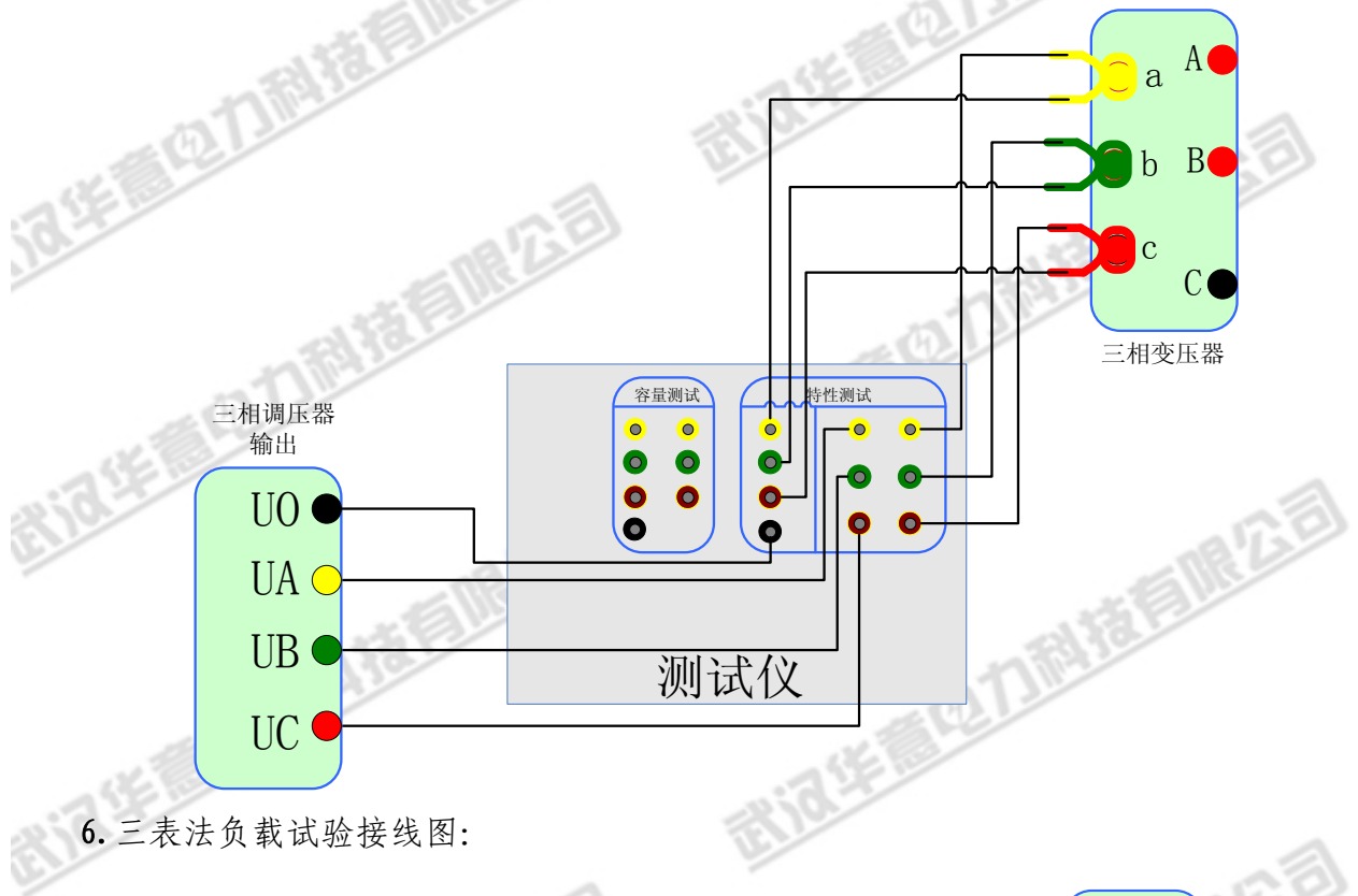
5. 三表法空载试验接线图:
