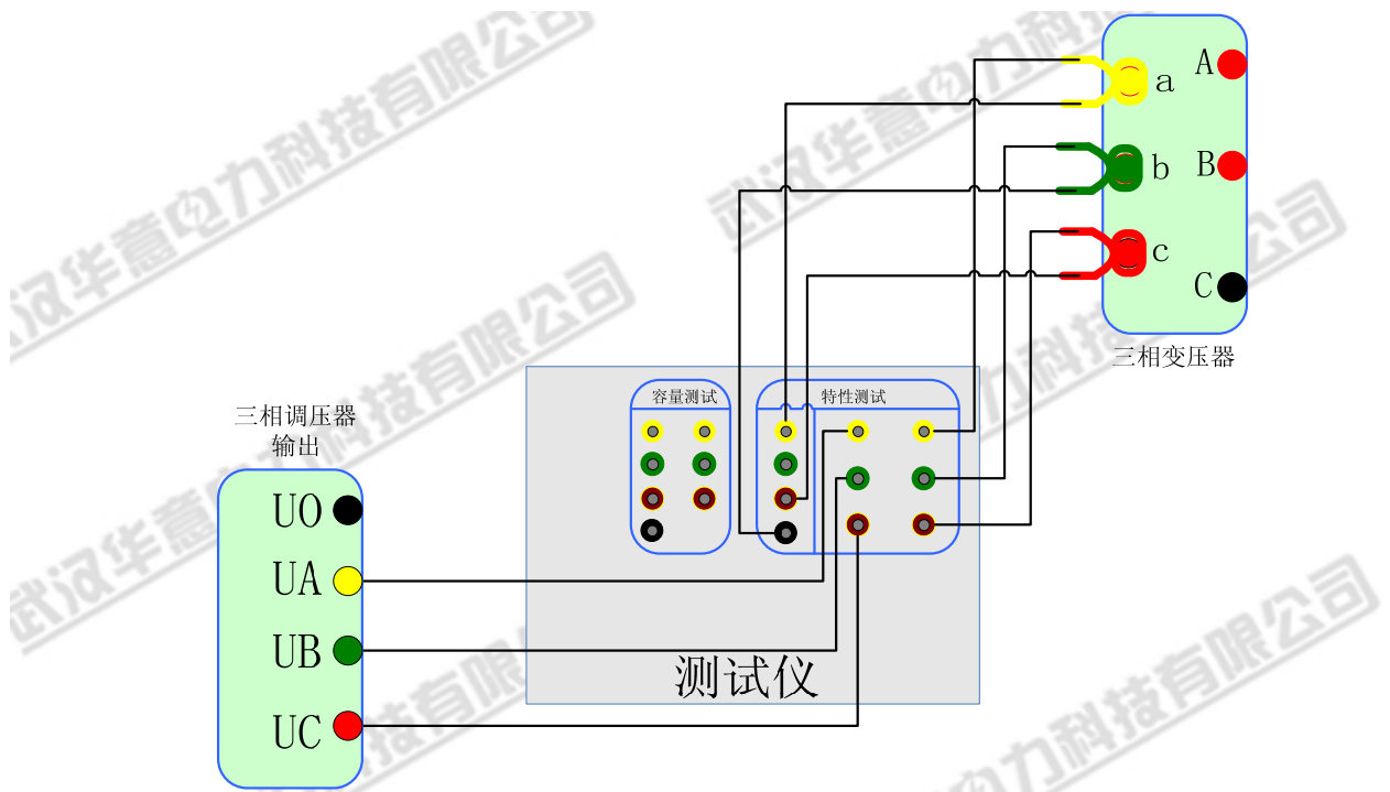
4. 双表法负载试验接线图:
