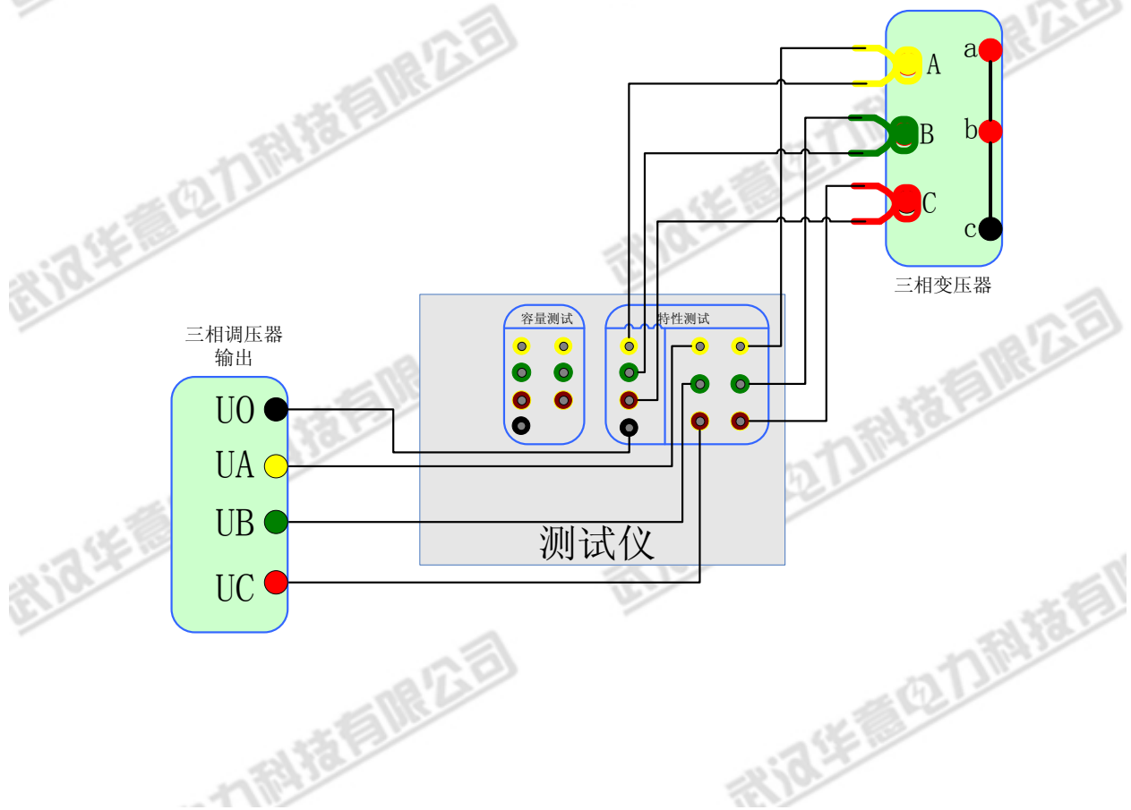
6. 三表法负载试验接线图:
