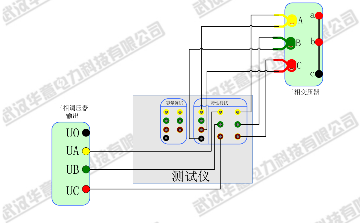
4. 双表法负载试验接线图:
