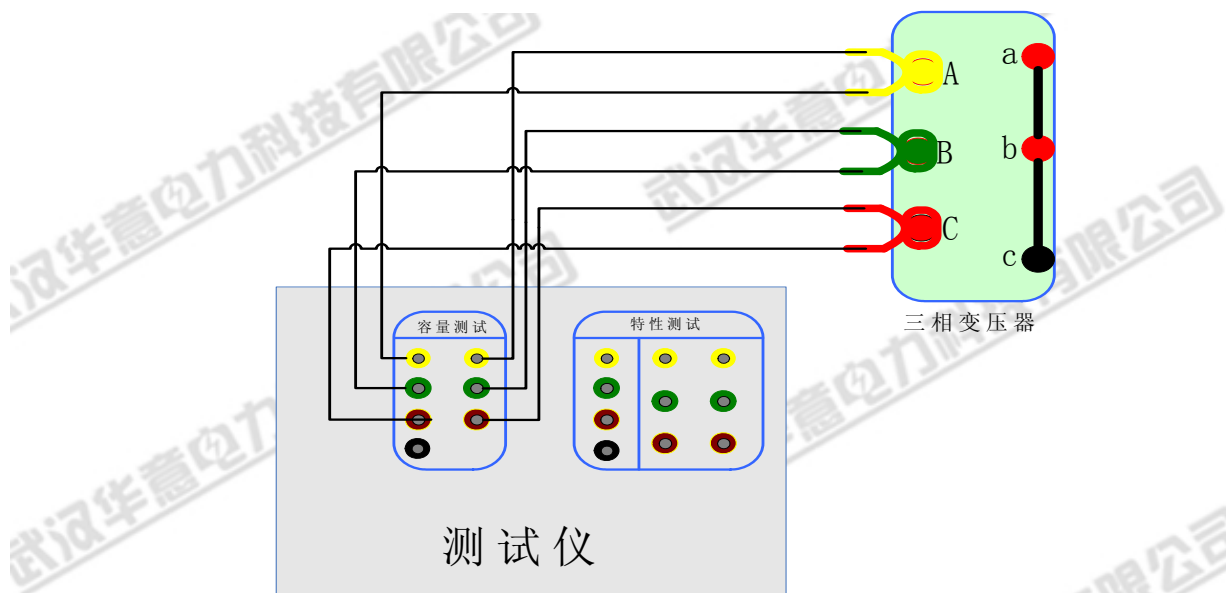
2. 单相变压器容量测试接线图:
