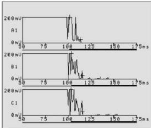
合闸动态电阻波形
