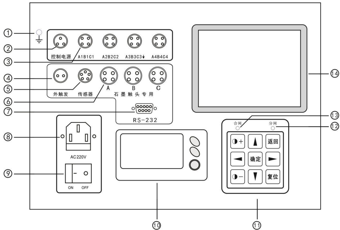
图 1 面板布局图
