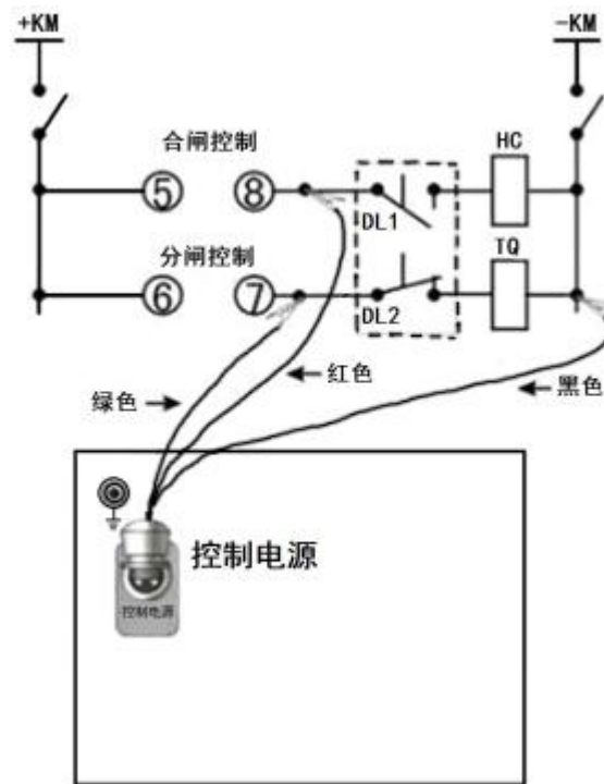
图 12 分合闸控制线接线图
