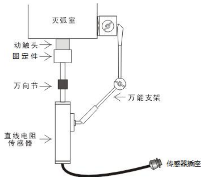
图 15 行程传感器安装示意图
