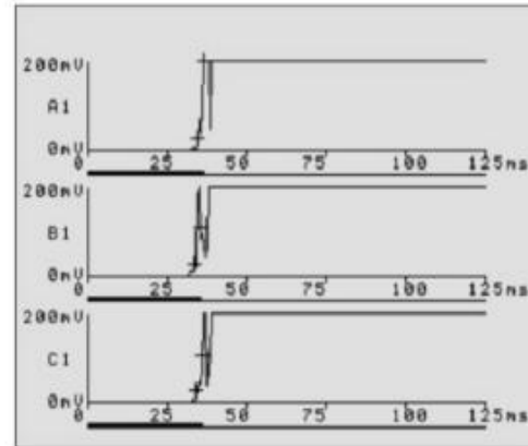
分闸动态电阻波形
